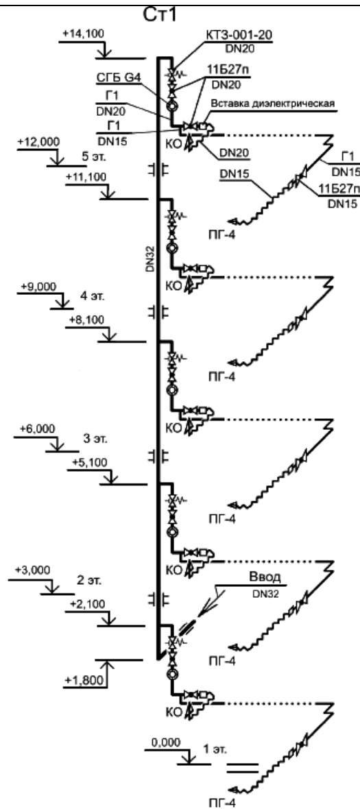
Рисунок Г.2 - Схема газоснабжения жилого дома
