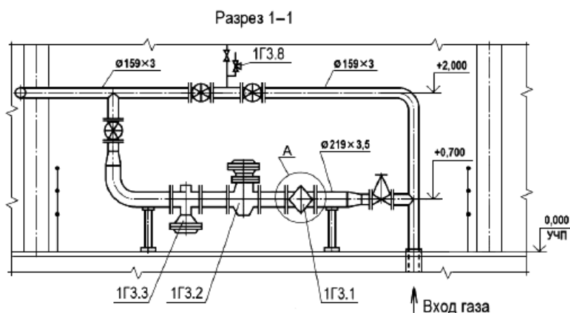
Рисунок Д.2 - Пример выполнения разреза
