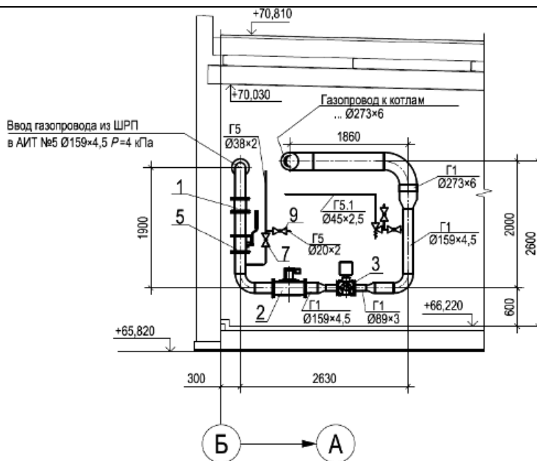
Рисунок В.2 - Пример выполнения разреза для котельной
