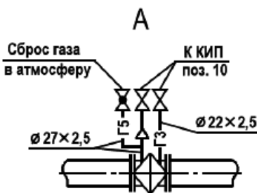
Рисунок Д.3 - Пример выполнения узла
