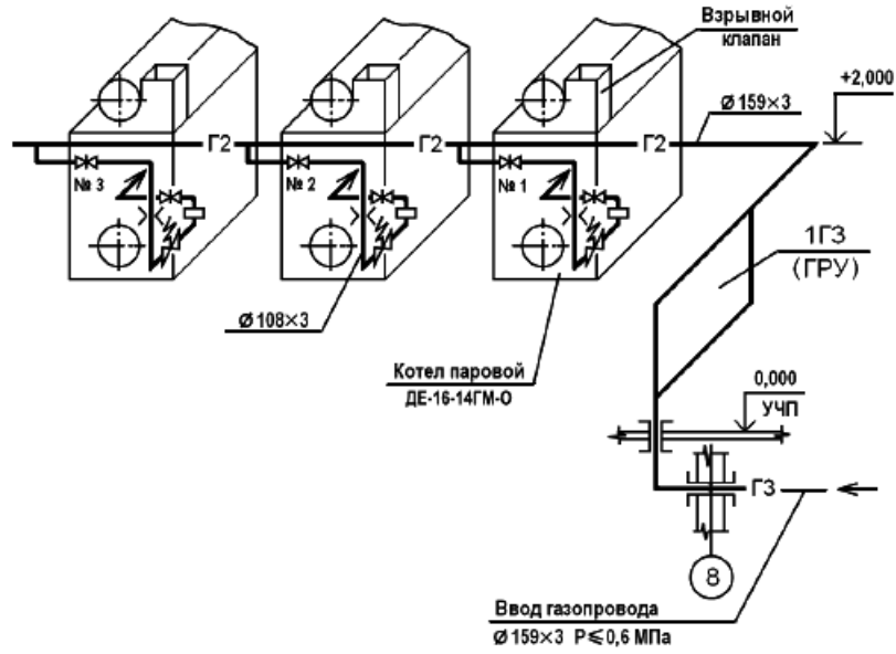
Рисунок Г.1 - Схема газоснабжения котельной
