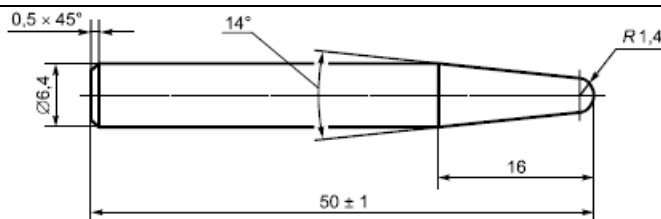
Рисунок Ф.2 - Размеры резца для выполнения прорезания
